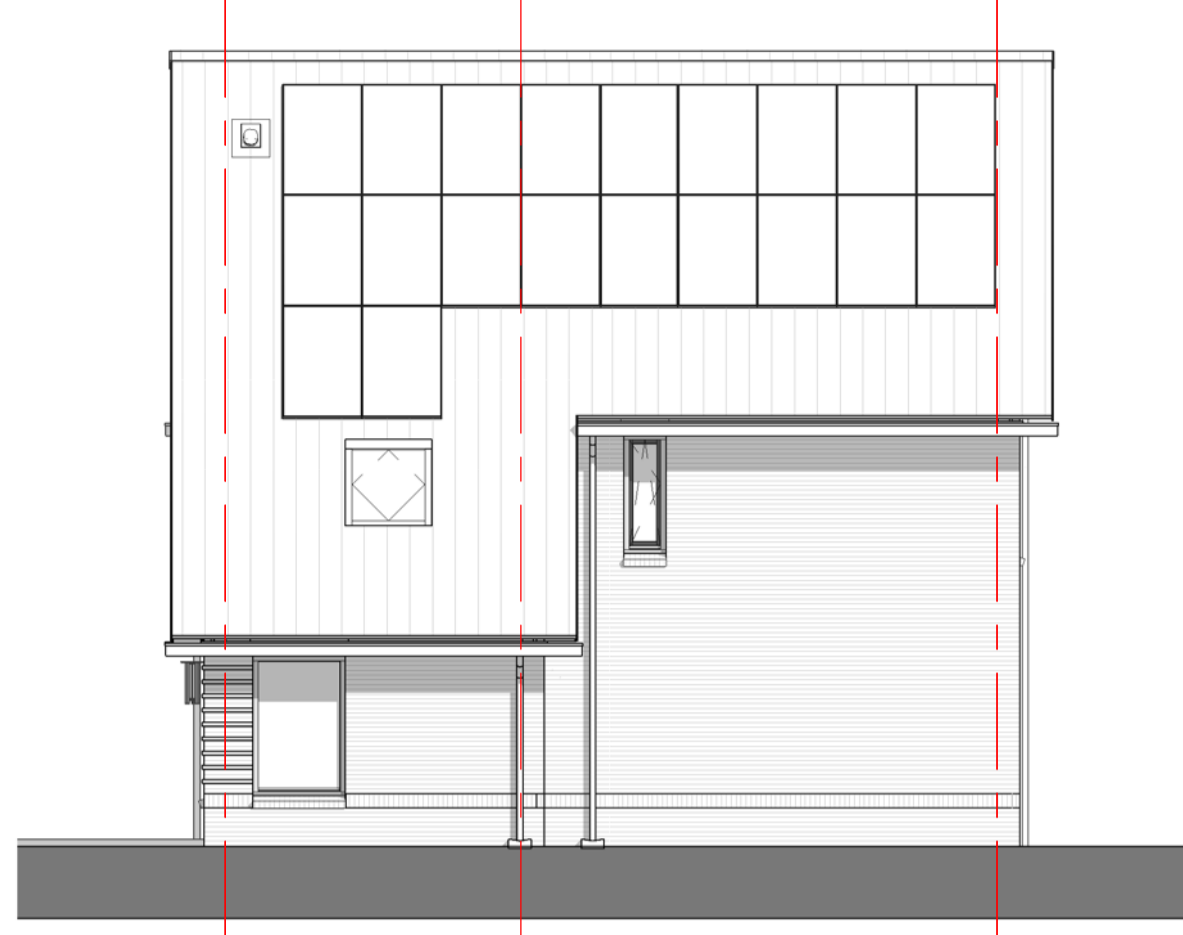
Rechter zijgevel Blok B
