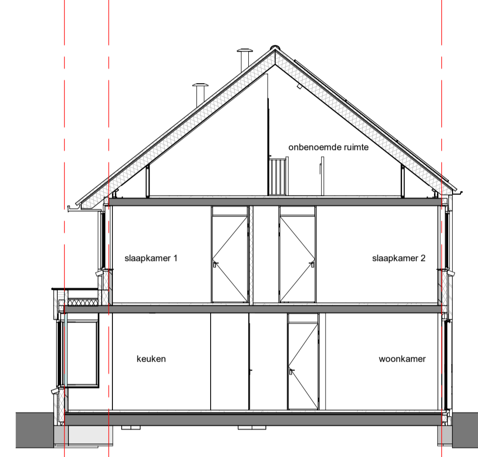
Doorsnede B-E
