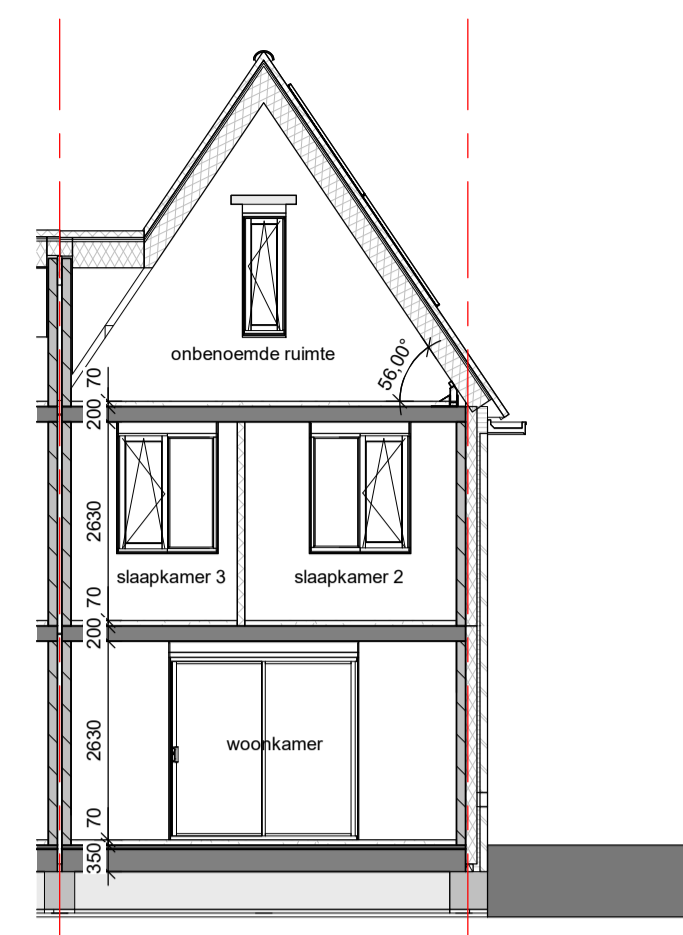
Doorsnede B-C
