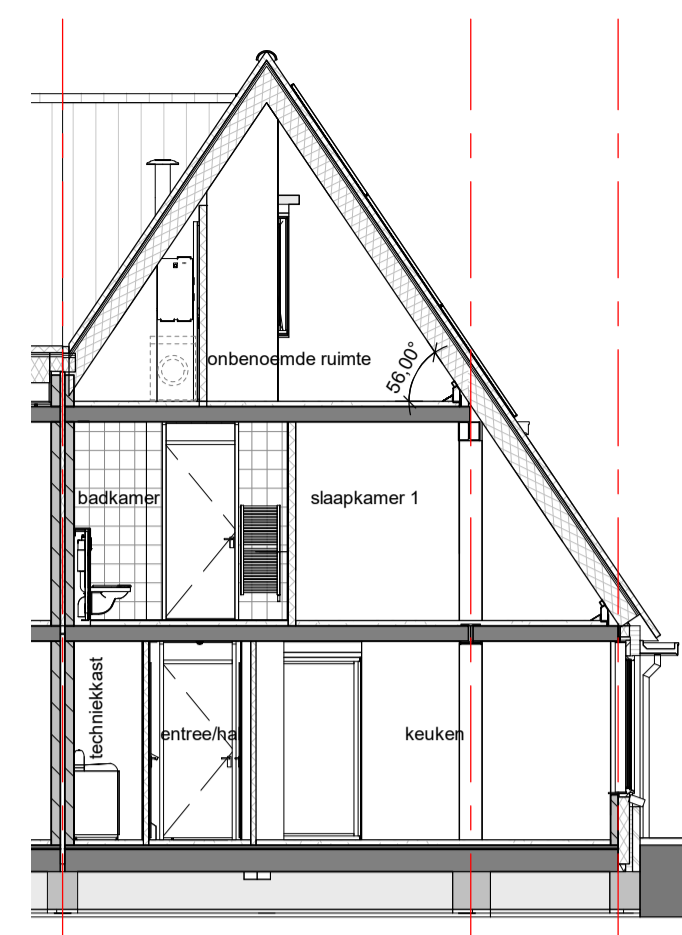
Doorsnede B-B
