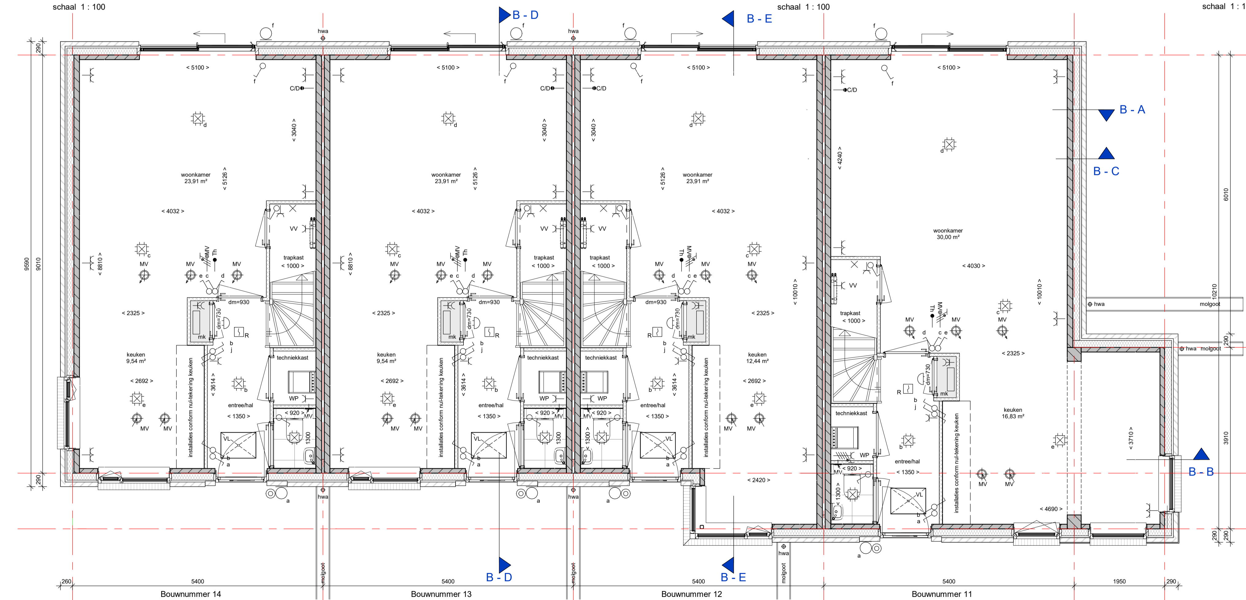
Begane grond Blok B
