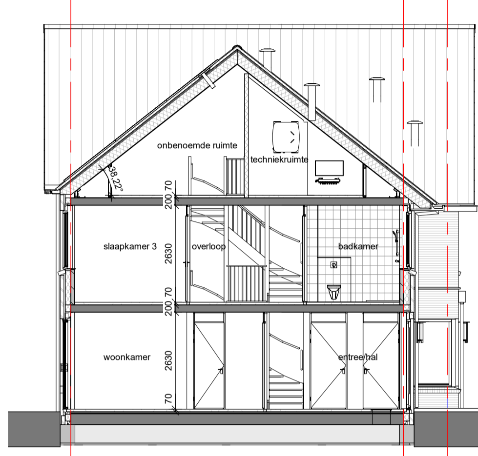
Doorsnede B-D
