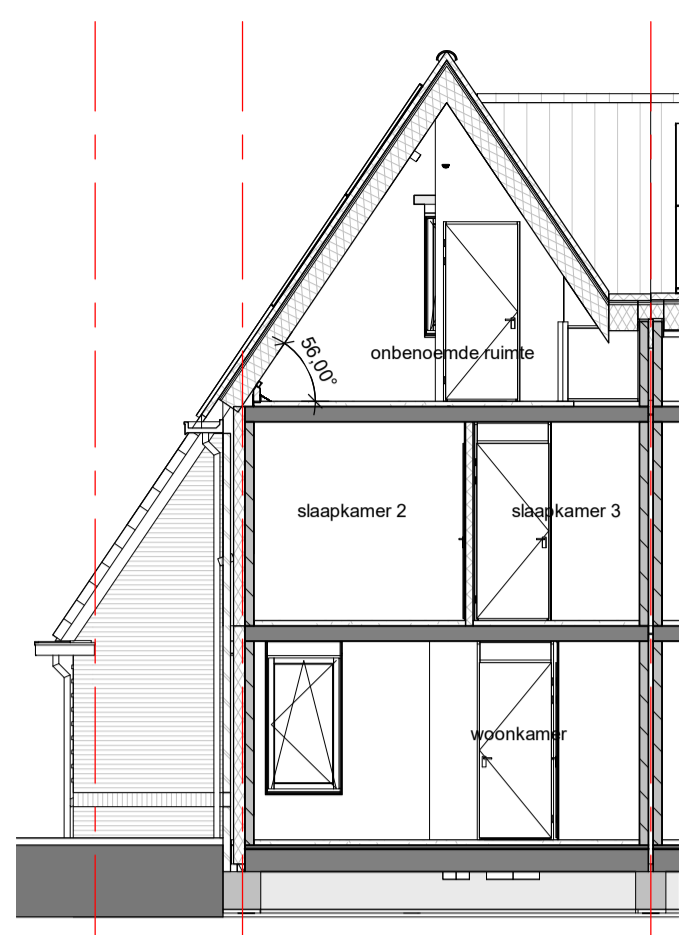
Doorsnede B-A
