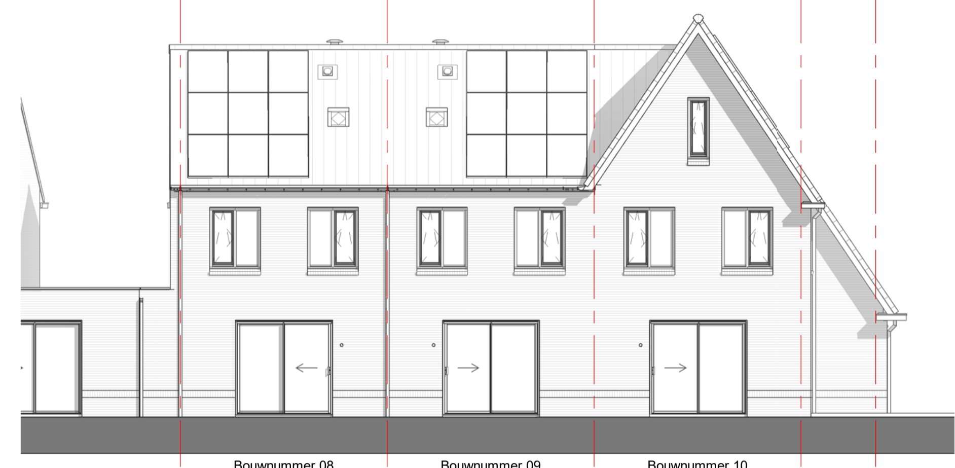
Achtergevel Blok A.2 schaal 1 : 100
