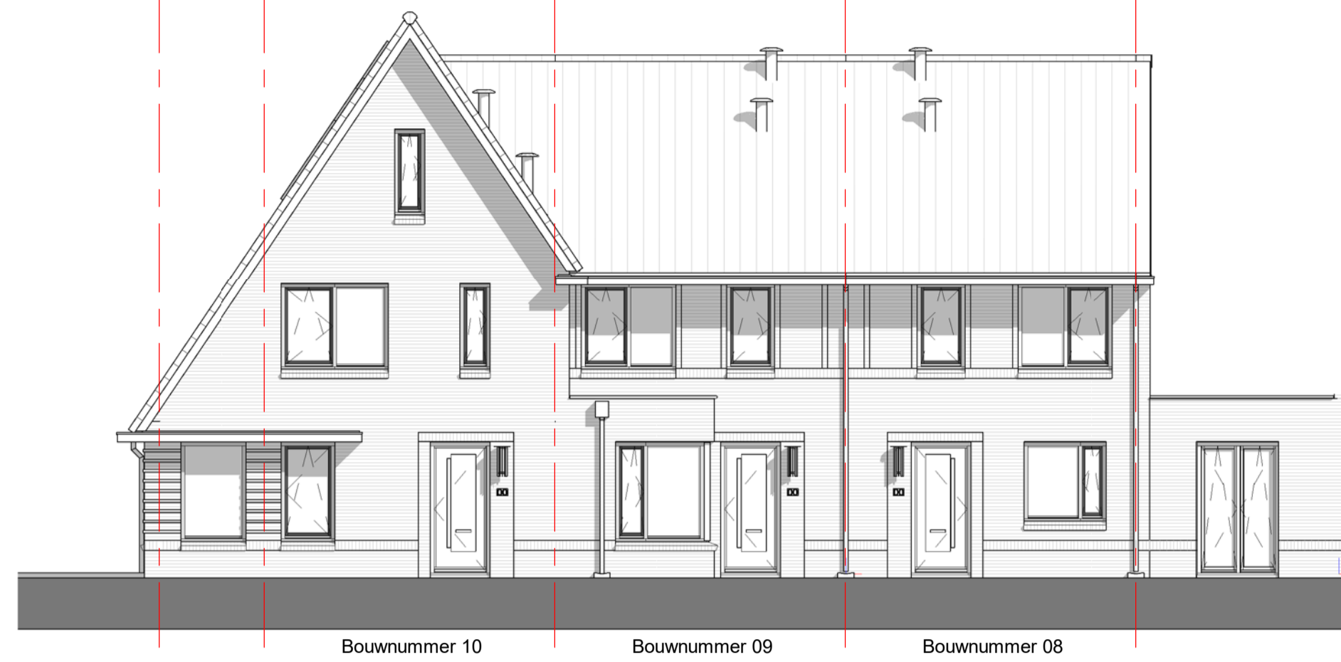
Voorgevel Blok A.2 schaal 1 : 100
