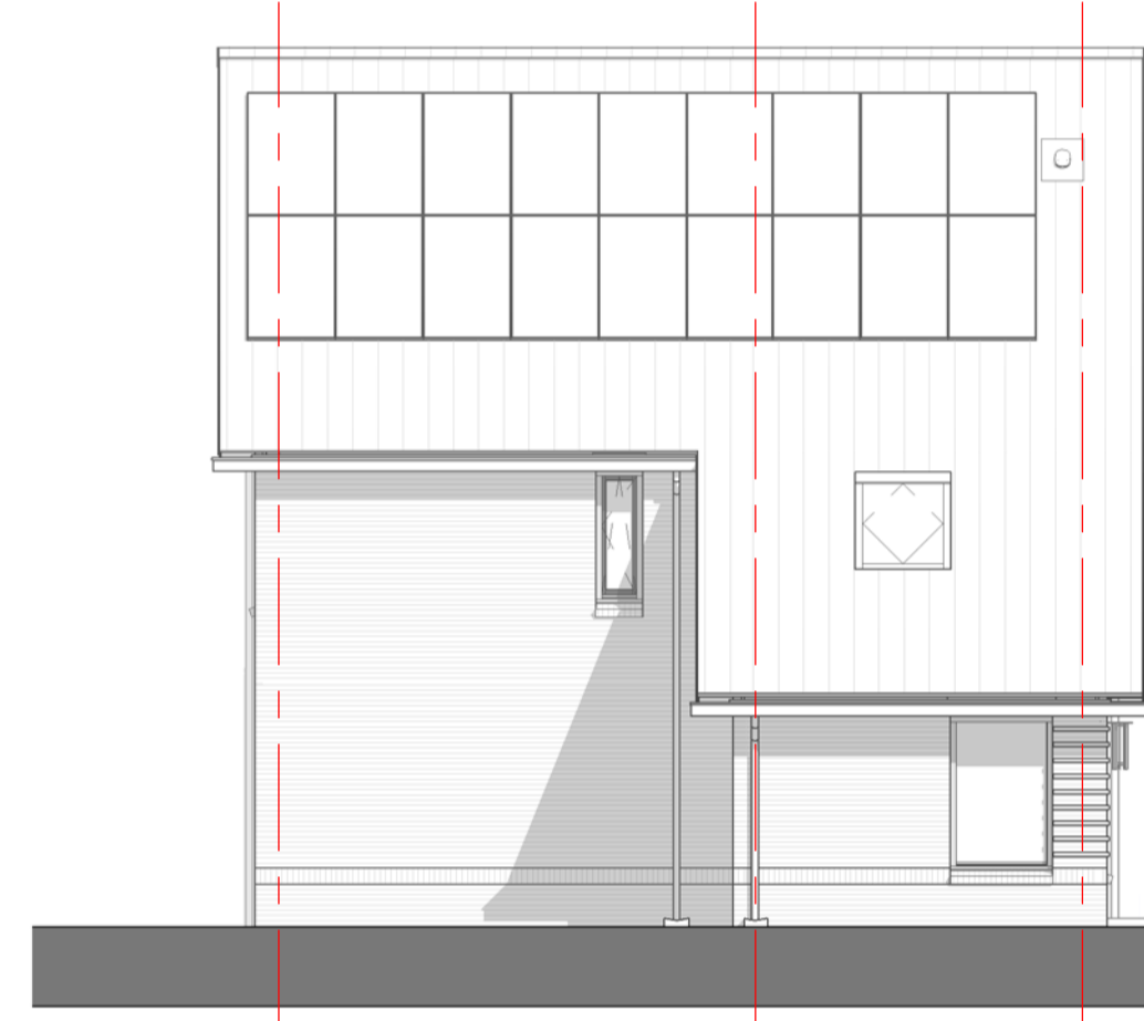
Linker zijgevel Blok A.2 schaal 1 : 100
