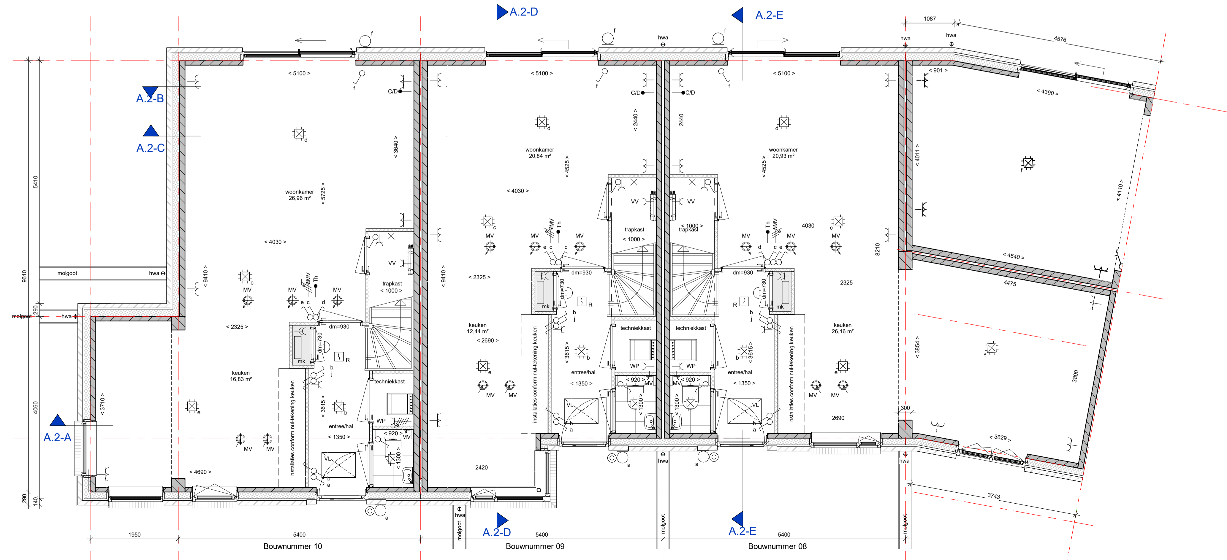
Begane grond Blok A.2 schaal 1 : 50
