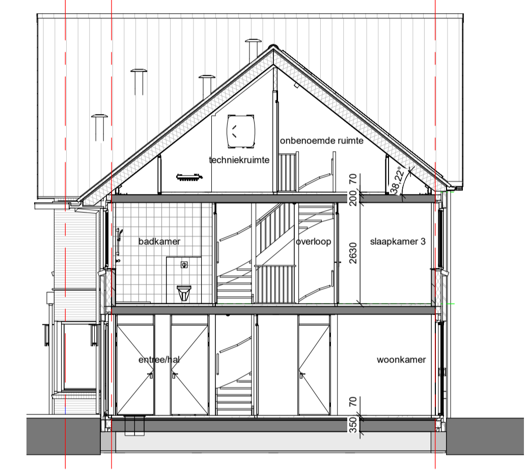
Doorsnede A.2-E schaal 1 : 100
