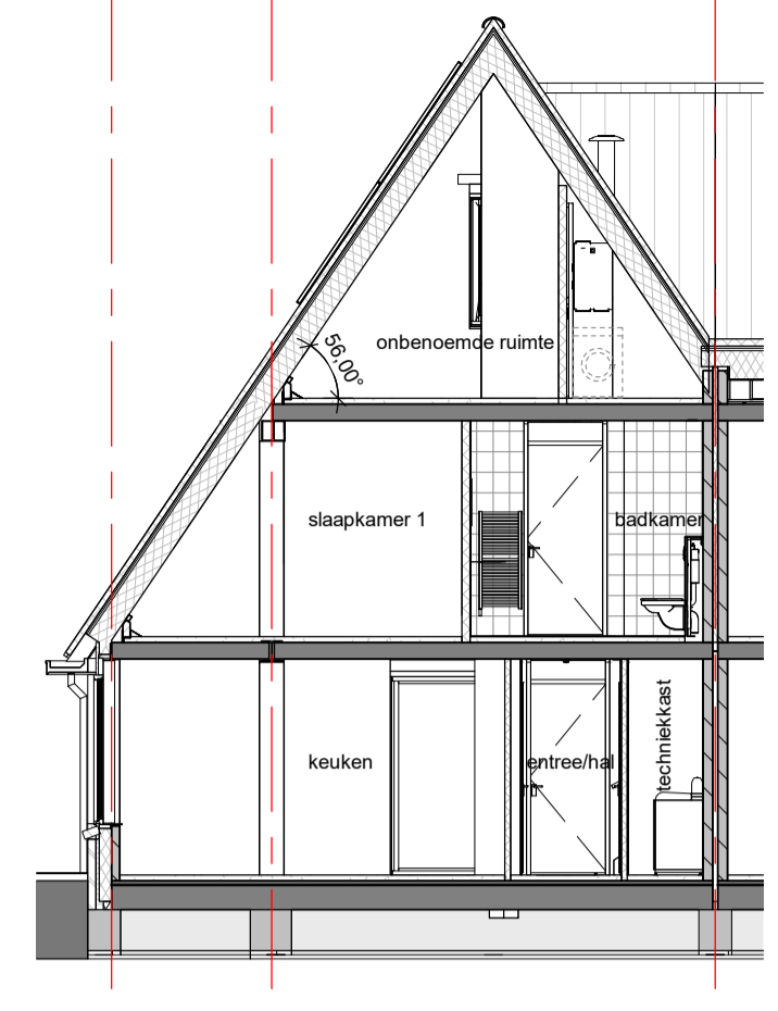
Doorsnede A.2-A schaal 1 : 100
