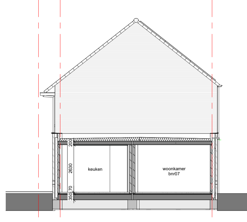
Rechter zijgevel Blok A.2 schaal 1 : 100
