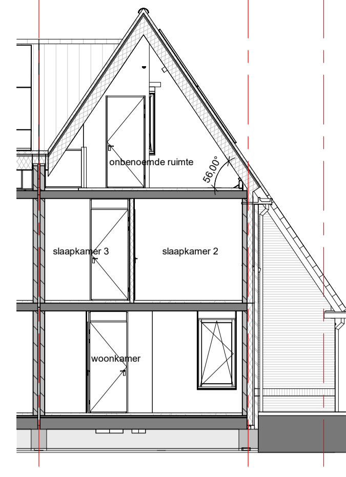
Doorsnede A.2-B schaal 1 : 100
