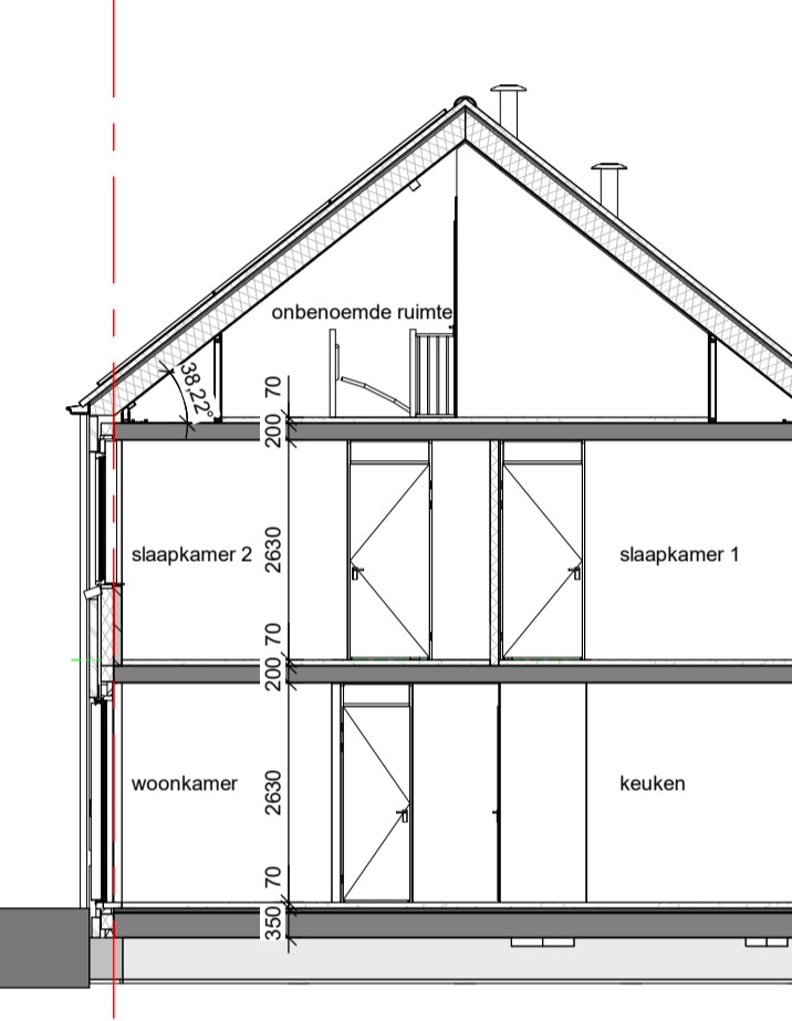
Doorsnede A.2-D schaal 1 : 100
