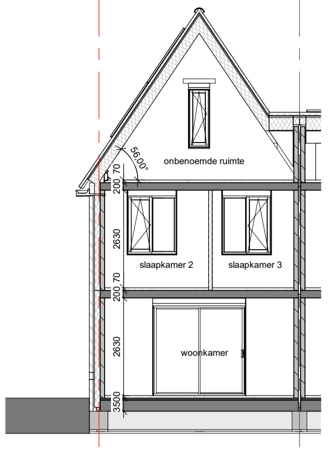
Doorsnede A.2-C schaal 1 : 100
