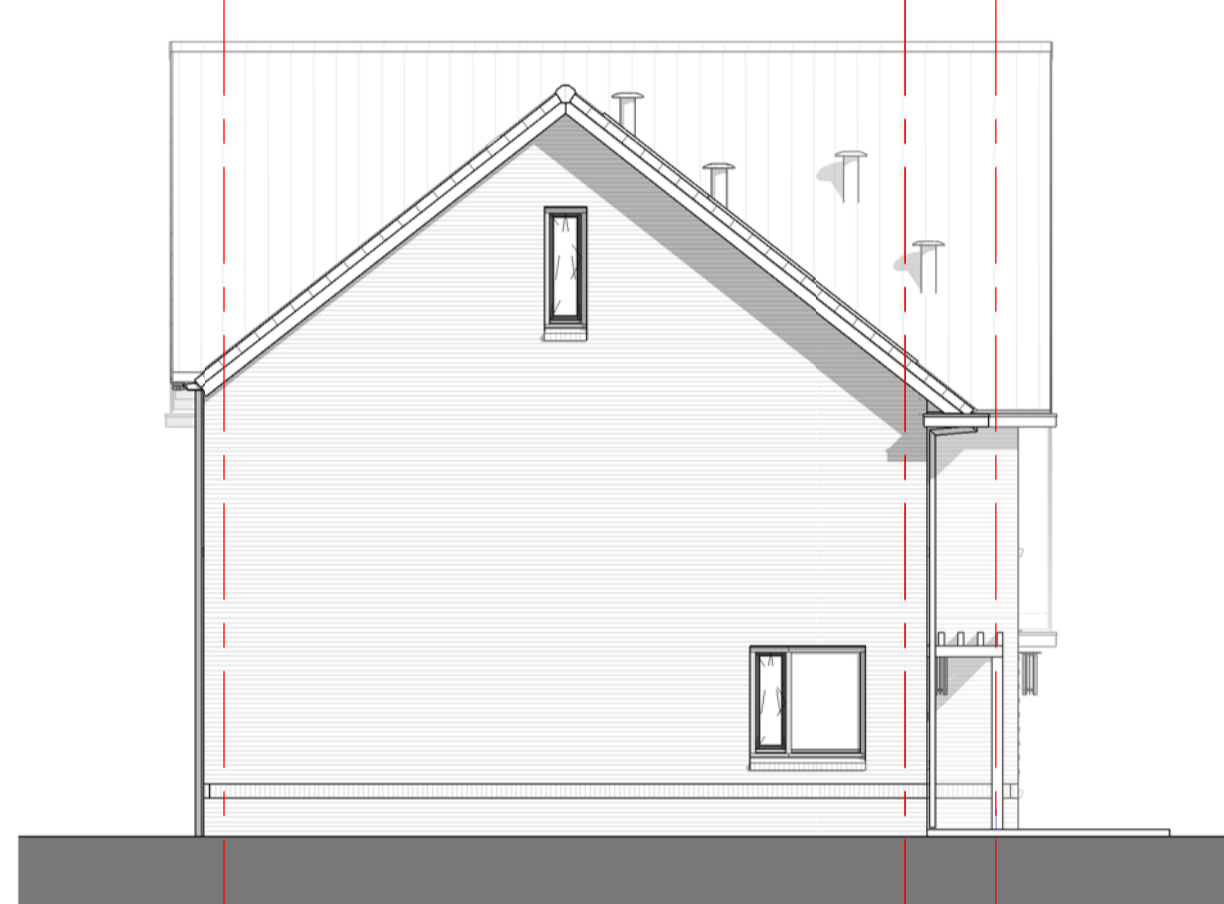
Linker zijgevel Blok C schaal 1 : 100
