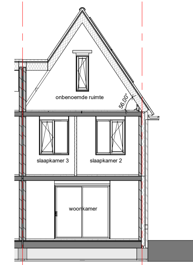
Doorsnede C-C schaal 1 : 100
