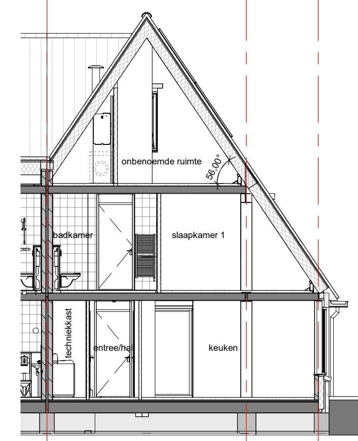
Doorsnede C-B schaal 1 : 100
