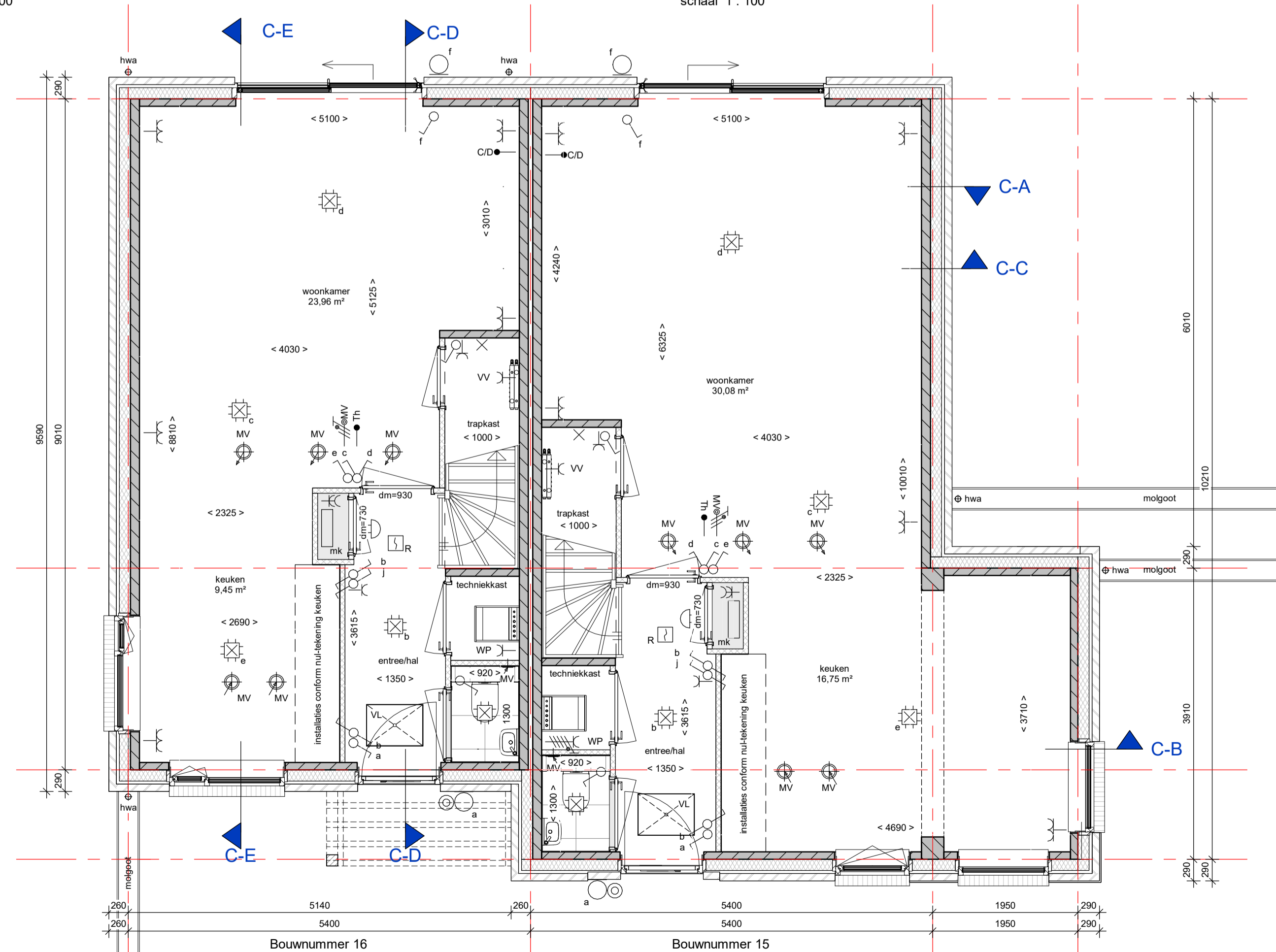
Begane grond Blok C schaal 1 : 50
