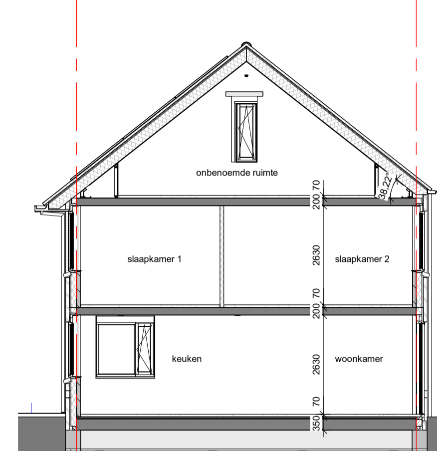
Doorsnede C-E schaal 1 : 100
