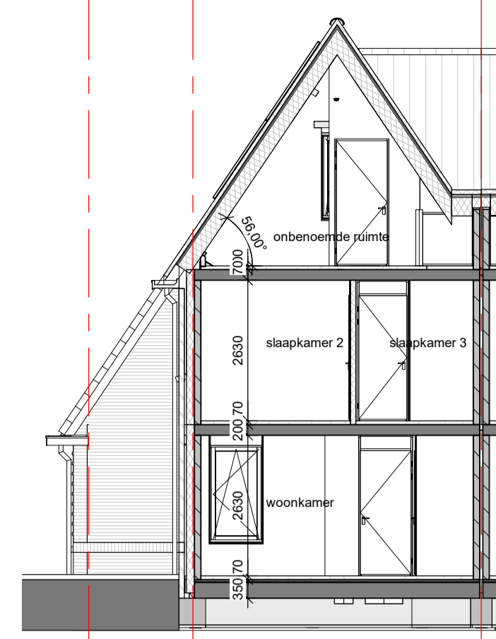
Doorsnede C-A schaal 1 : 100
