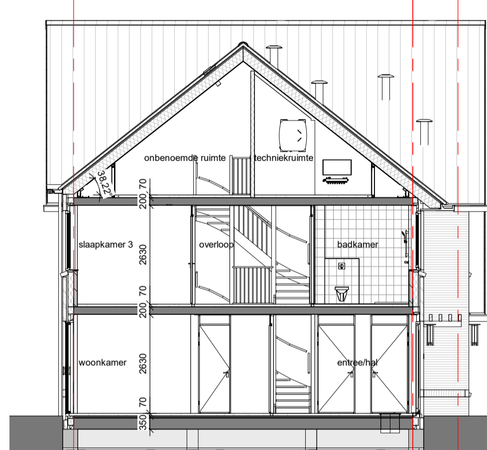
Doorsnede C-D schaal 1 : 100
