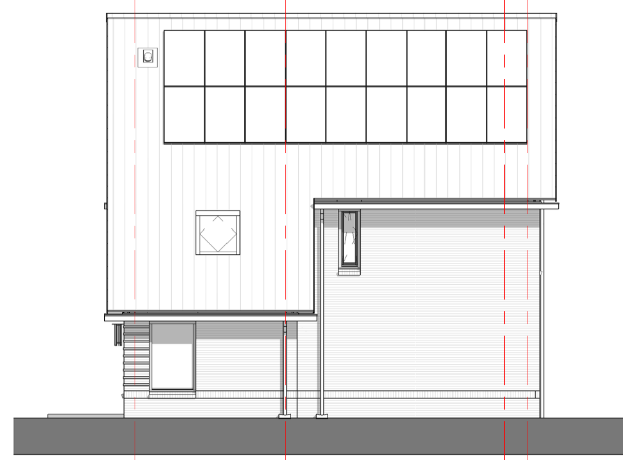
Rechter zijgevel Blok C schaal 1 : 100
