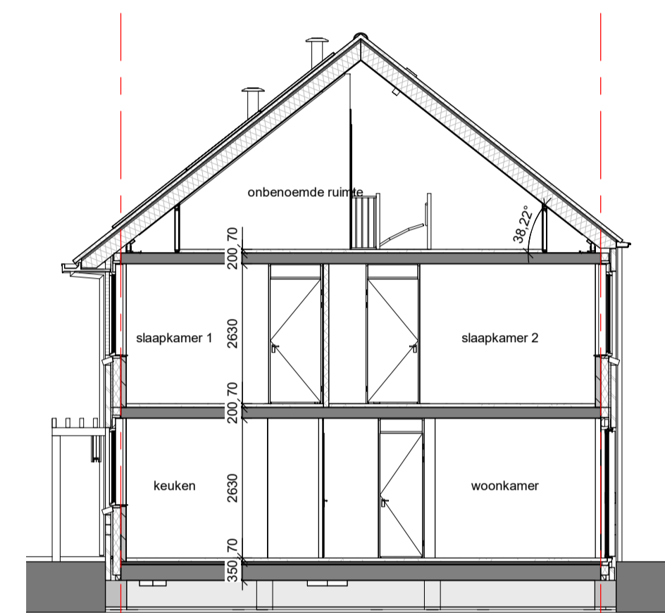
Doorsnede E-B
