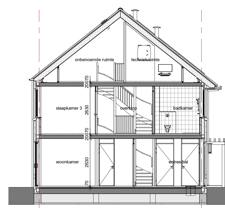
Doorsnede E-A
