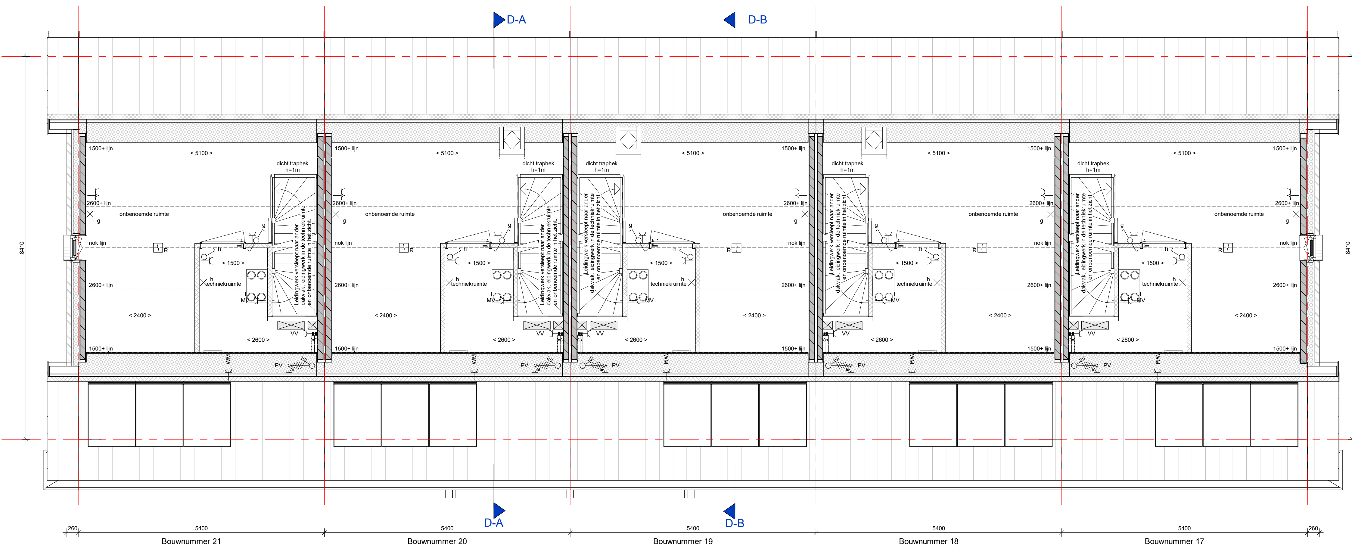
2e verdieping Blok D
