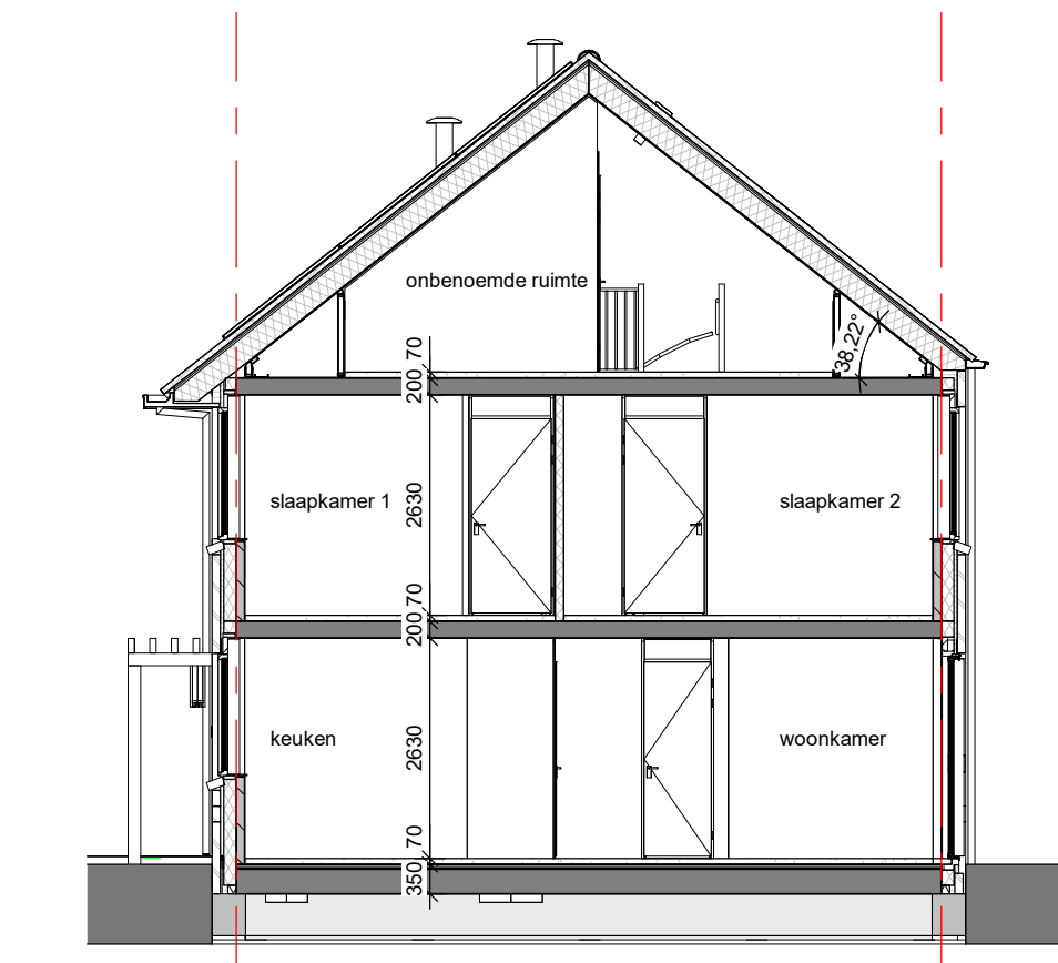
Doorsnede D-B
