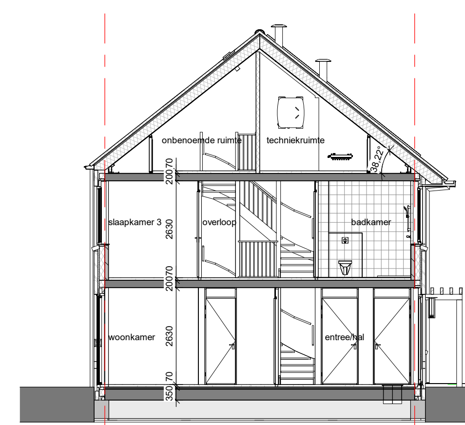
Doorsnede D-A
