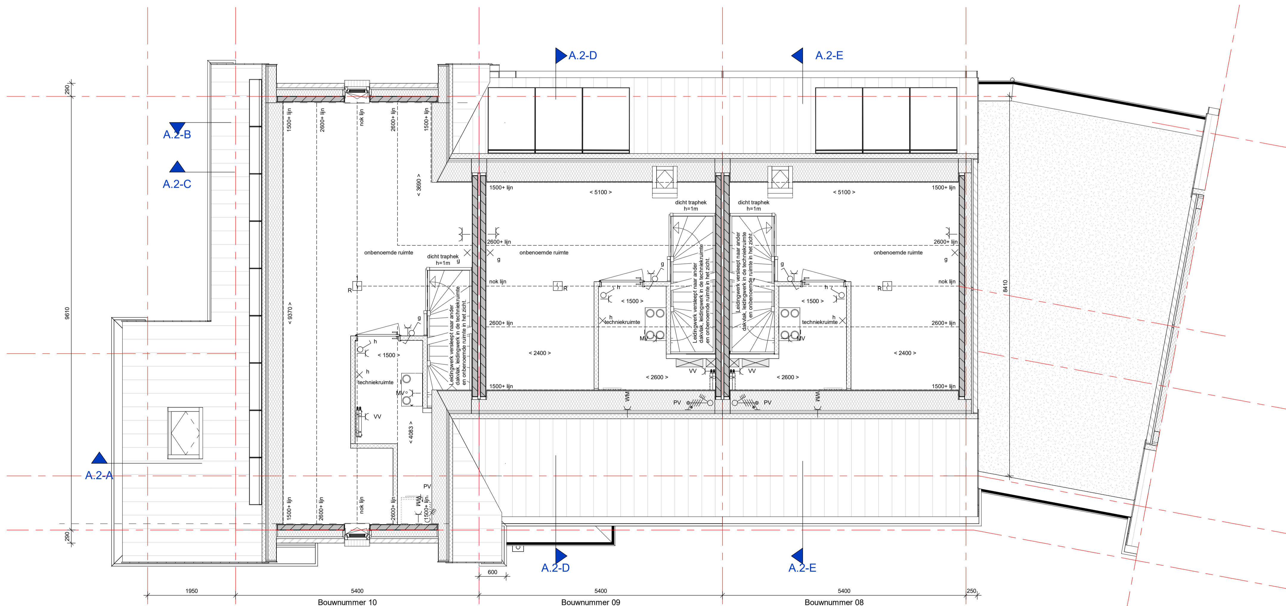
2e Verdieping Blok A.2
