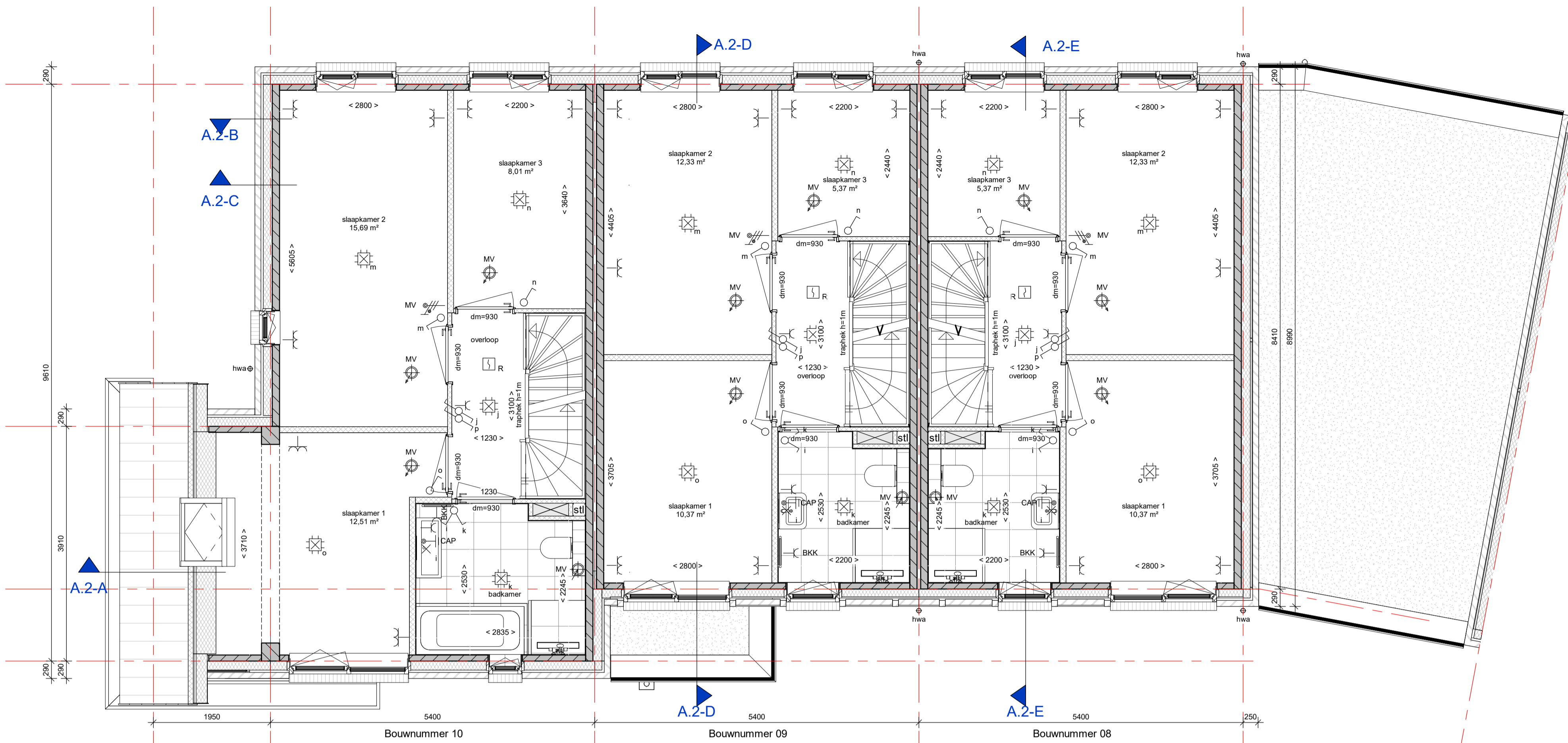
1e Verdieping Blok A.2
