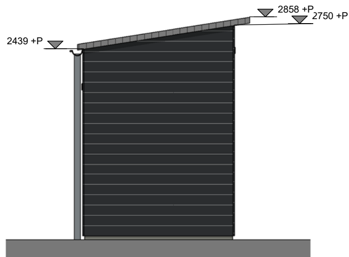
Achtergevel Berging
