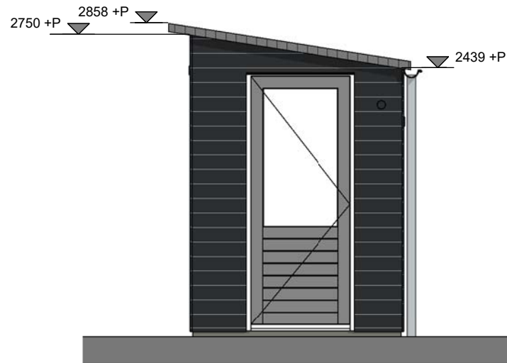
Voorgevel Berging
