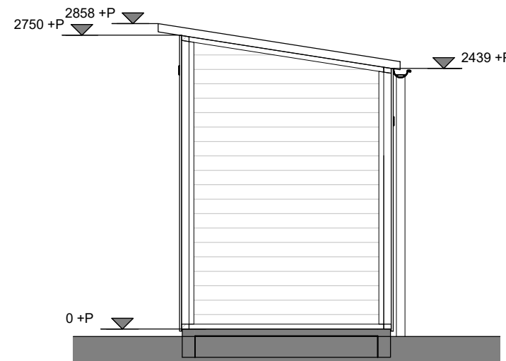
Doorsnede A3
