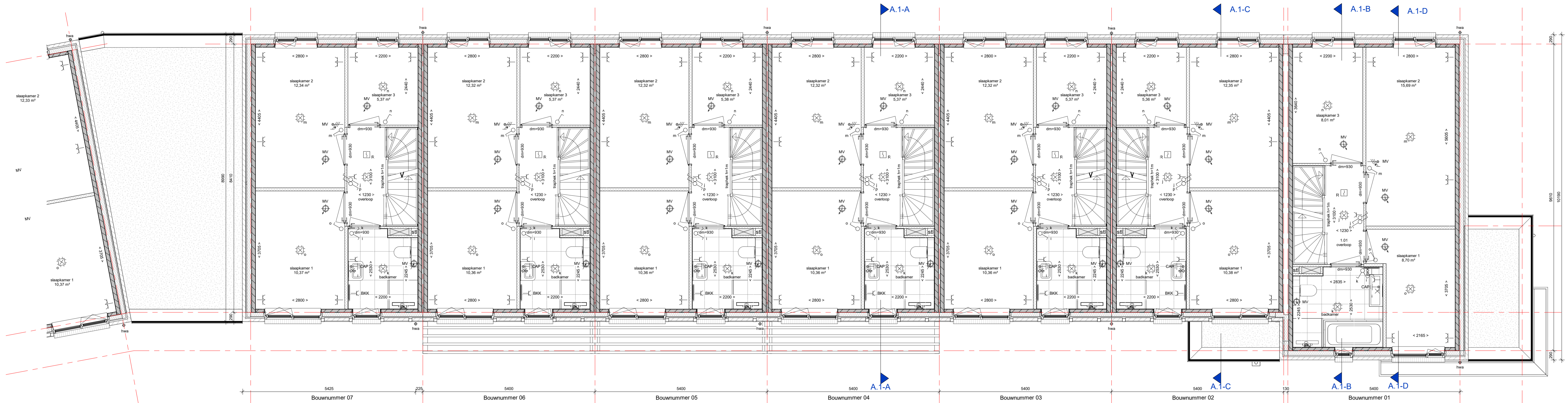
1e Verdieping Blok A.1 schaal 1:50
